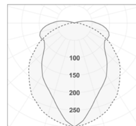
Version 1 lampe Réflecteur intensif
