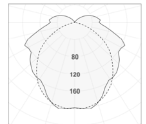
Version 2 lampes Réflecteur extensif
